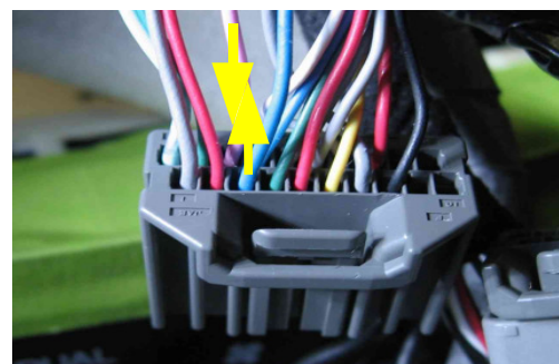
20 poliger Stecker an der Rückseite des Audio Systems
